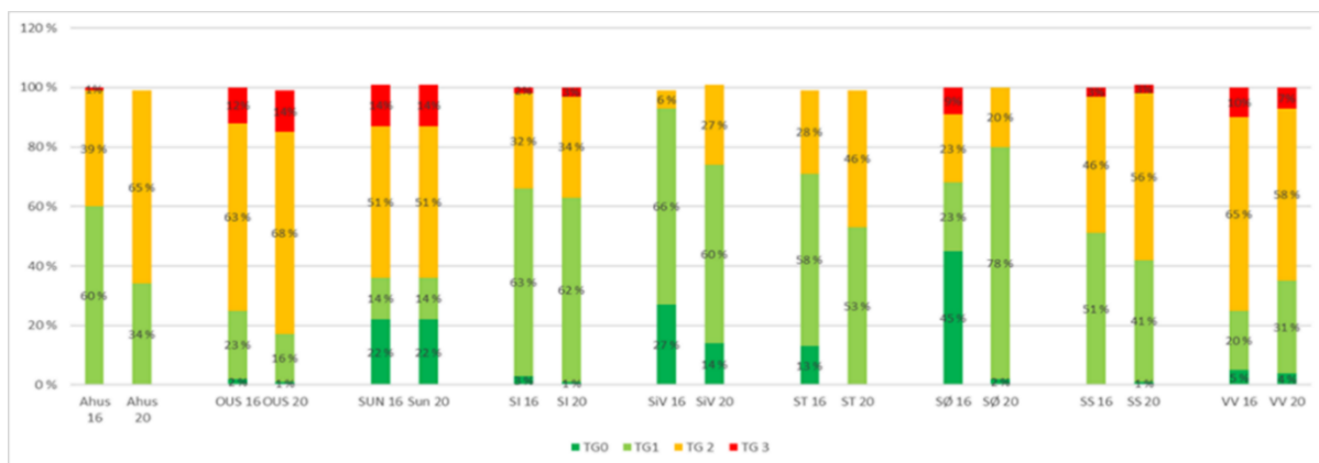
Samlet vektet tekniske tilstandsgrad (VTTG) 2020: Ahus 1,6 OUS 1,85 SUN 1,47 SI 1,41 SIV 1,17 ST 1,51 SØ 1,16 SS 1,65 VV 1,64 Figur 10: Tilstandsgrad for bygg i 2020 for helseforetakene (merk: 2020 er siste foreliggende oppdatering).
